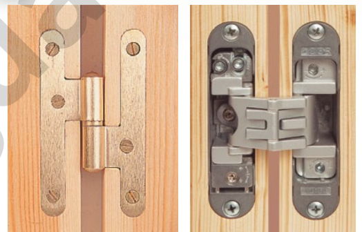
Acabados perfectos en la realización de encajes. Colocación de bisagras invisibles en una sola operación y sin cambiar la plantilla.
