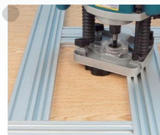
El proceso de fresado se realiza con gran estabilidad y eficacia.
