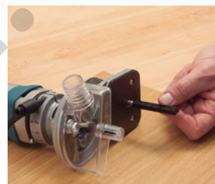
Dispositivo de guiado para el perfilado de esquinas alojado en la base cuando no se usa. Su colocación es muy rápida y sencilla.
