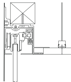
SIN DINTEL / WITHOUT LINTEL
