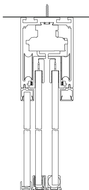
CON VIDRIO FIJO / WITH FIXED GLASS
