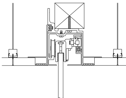
SIN DINTEL / WITHOUT LINTEL
