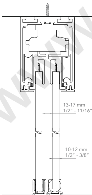
SIN VIDRIO FIJO / WITHOUT FIXED GLASS
