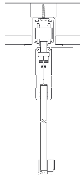
EMPOTRADO / RECESSED PERFIL TOP / TOP TRACK
