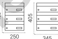
H2000-G3 Fondo 270 H2100-G3 Fondo 270 H2200-G3 Fondo 365
