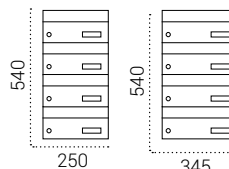
H2000-G4 Fondo 270 H2100-G4 Fondo 270 H2200-G4 Fondo 365
