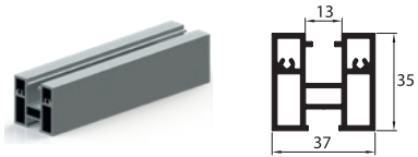
Perfil horizontal
