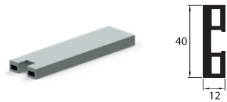
Perfil vertical
