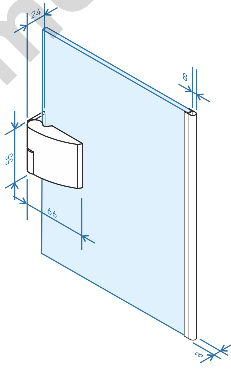
bisagra a pared con cierre perfil burbuja
