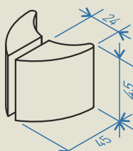
tirador media luna (opcional sin incremento)
