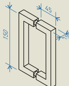
asa tirador (opcional 50€)
