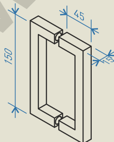
asa tirador (de serie)
