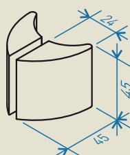
tirador media luna (opcional 55€)
