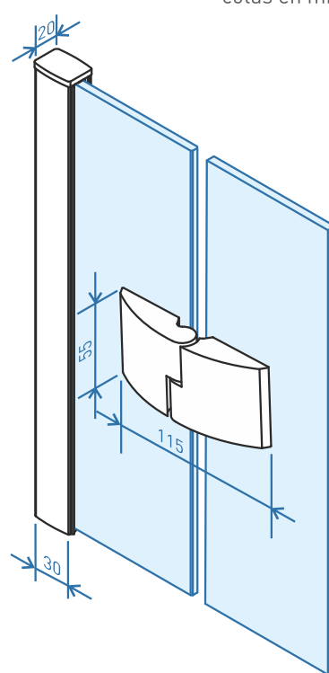
perfil con regulación en pared y bisagra doble
