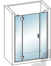
frontal de ducha 1 puerta abatible 180° 2 fijos frontales
