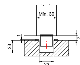
Montaje a suelo de guía inferior + guiador
