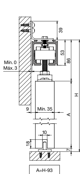
Montaje a pared accesorios pletina
