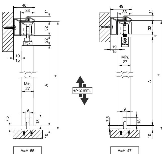
Guía Star pletina + Perfil Separador
