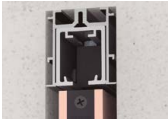
Conjunto Perfil Funda FT XL+ STAR XL
