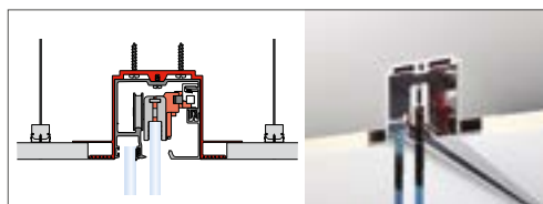
Instalación oculta falso techo
