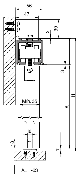
Montaje a pared accesorios retráctil
