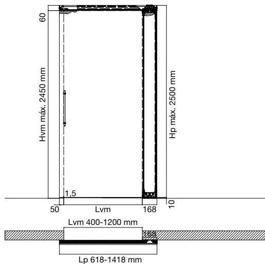
Sin guías ni guidores en el suelo
