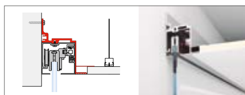
Instalación a pared
