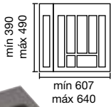
Módulo 70 Cubterero M-60 + bandeja de 110 mm.
