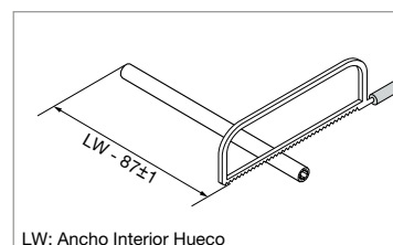
LW: Ancho Interior Hueco
