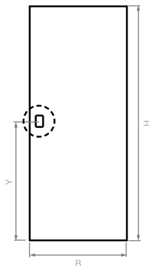
Fresado de las hojas
